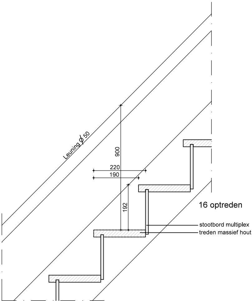
DETAIL D1 detail nieuwe dichte trap
