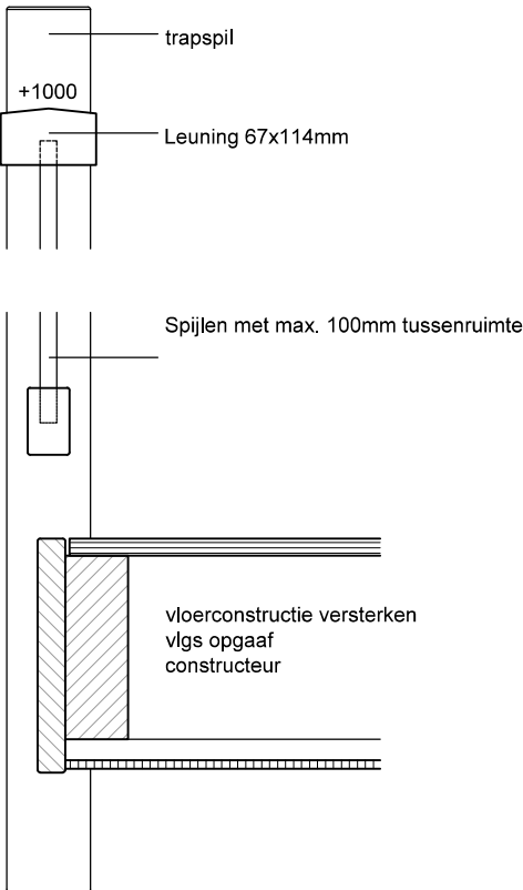
DETAIL D2 vloerafscheiding
