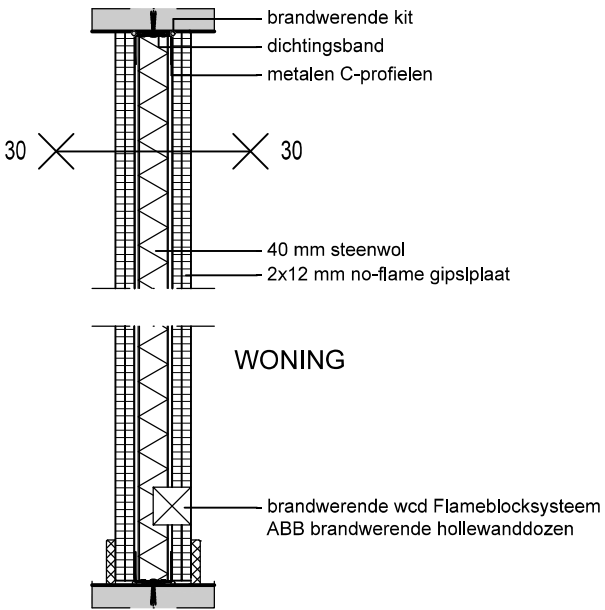
DETAIL D3 Woningscheidende wand 30 min. WBDBO
